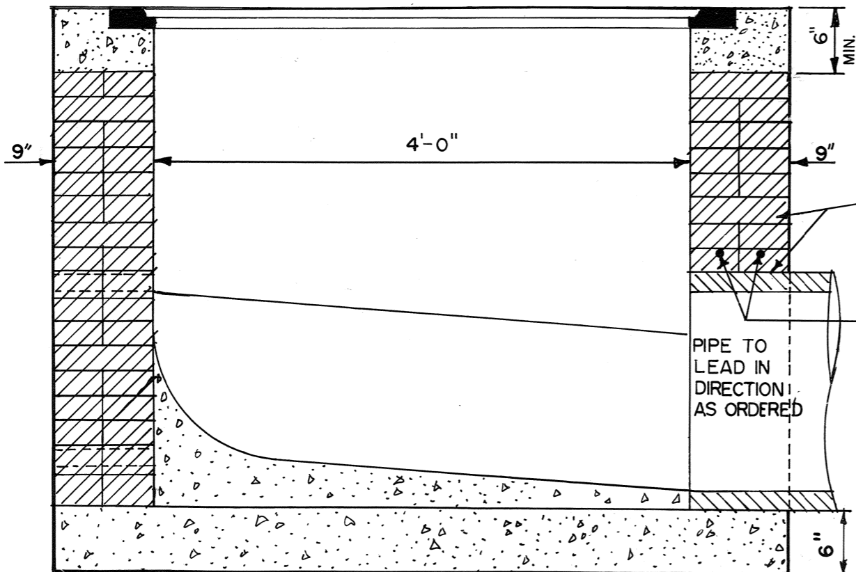
LONGITUDINAL SECTION
